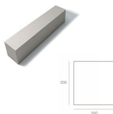
Bordillo Rigola 20 X 20
